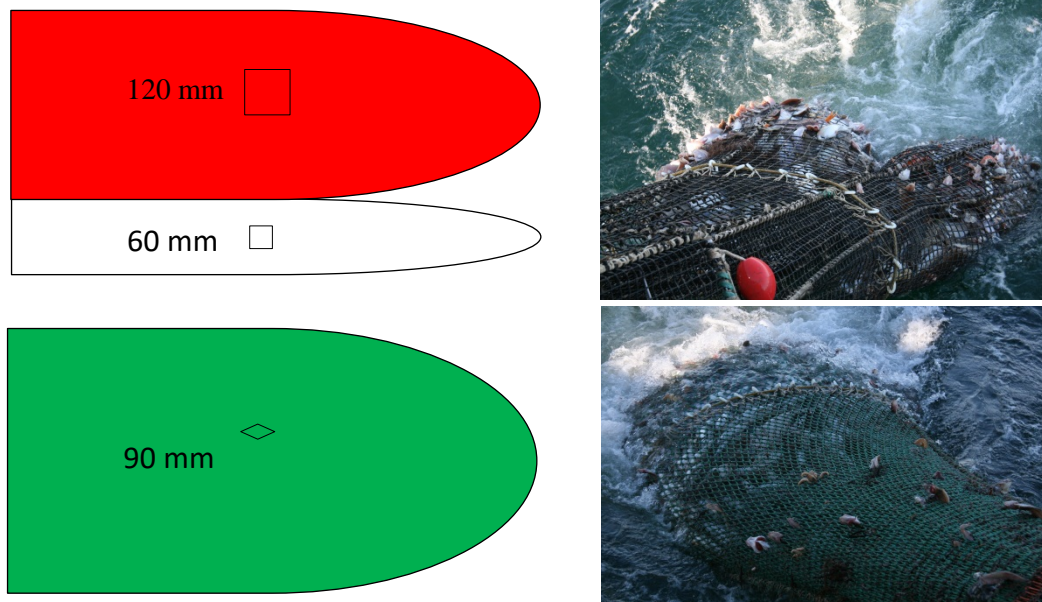
Figur 4. Venstre: Farvekoder tildelt fangst fra fiskeposen (rød) og hummerposen (hvid) i den horisontaldelte fangstpose, samt standardposen (grøn). Højre: De to fangstposer under fiskeri.
