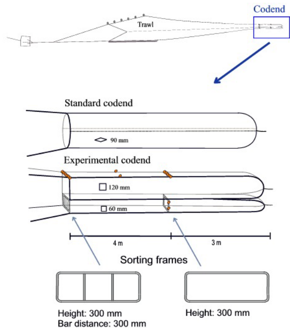
Figur 3. Udvikling og produktion af den horisontaldelte fangstpose i samarbejde med vodbinder og fiskeskipper (venstre). Skematisk illustration af standardposen og det endelige design på den horisontaldelte (eksperimentelle) fangstpose.
