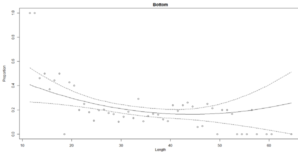
Figur 20. Den fuldt optrukne linje viser den estimerede fangstandel af kuller i hummerposen ved anvendelse af Model 3 (se Appendix B). 95% konfidencegrænserne er indikeret med de stiplede linjer. De observerede værdier er vist som åbne cirkler. p_{l,c=bottom} .
