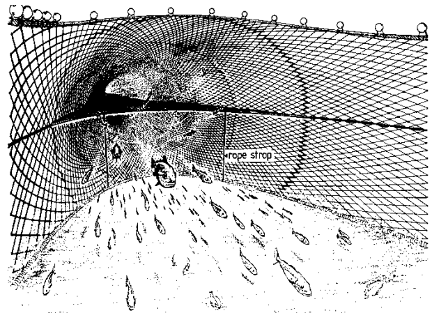
Figur 2. Horisontaldelt redskab hvor vertikal delingen starter fremme i trawllåbningen (Main og Sangster 1985).
